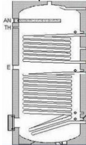
Solarspeicher
